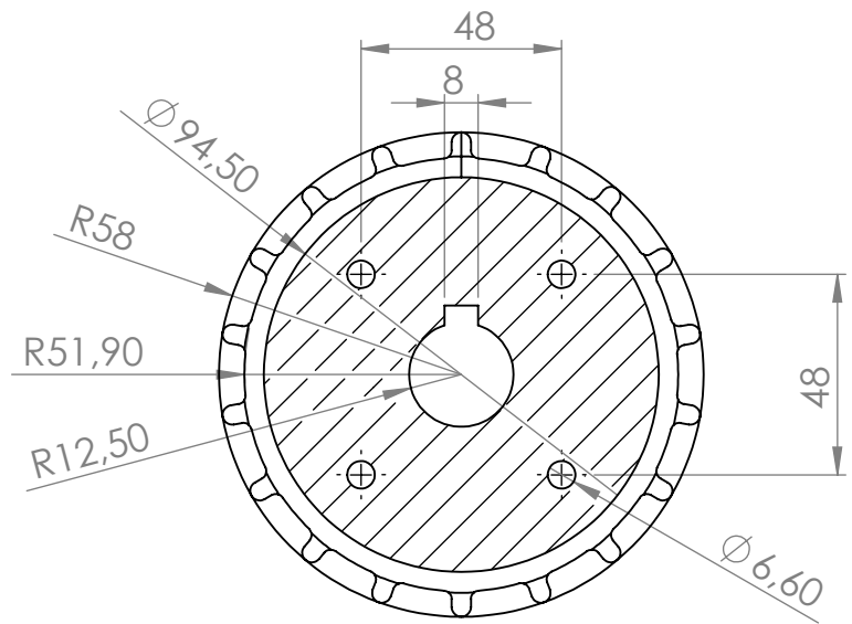
KESIT A-A
